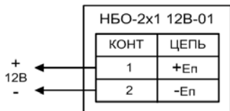
Рис.1 Схема подключения.
