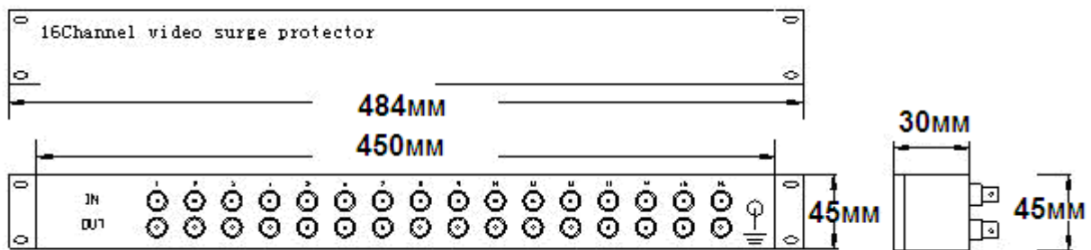
Рис.2 Габаритные размеры SP-C8C, SP-C16C, SP-C24C
