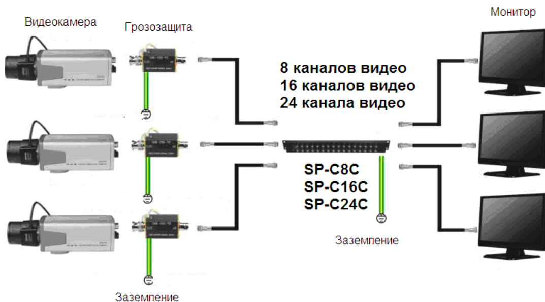
Рис.3 Подключение SP-C8C, SP-C16C, SP-C24C
