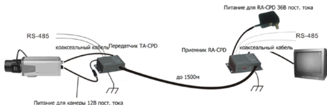
Рис.4 Схема подключения передатчика TA-CPD и приемника RA-CPD
