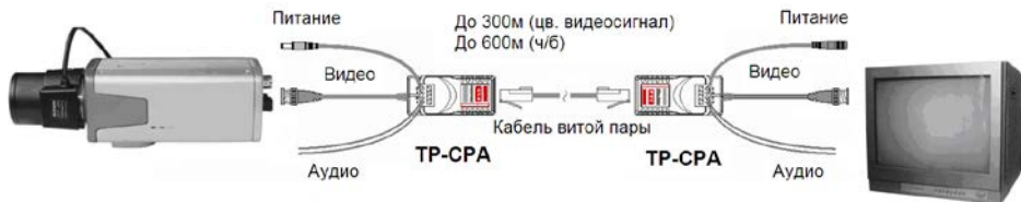
Рис.2 Схема подключения TP-CPA
